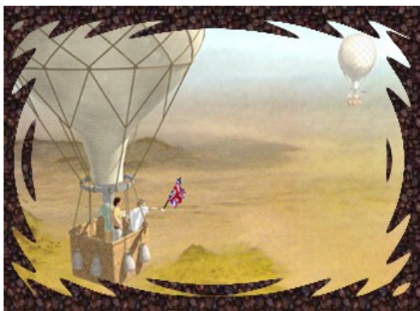
Filtro Distorsión-->Ondas
